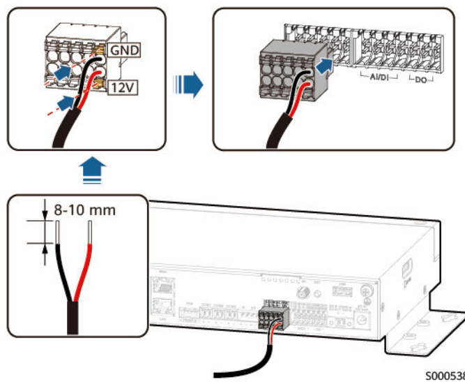
Abbildung 4-13 Anschließen eines Ausgangstromkabels
