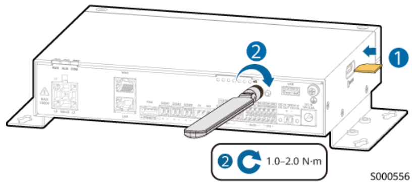
Abbildung 4-19 Installieren einer SIM-Karte und einer 4G-Antenne
