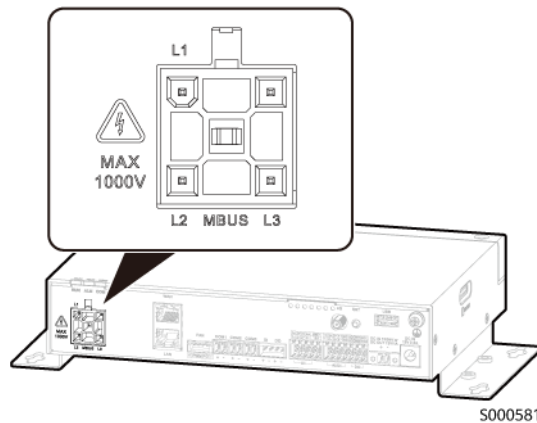
Abbildung 2-7 MBUS-Anschluss
