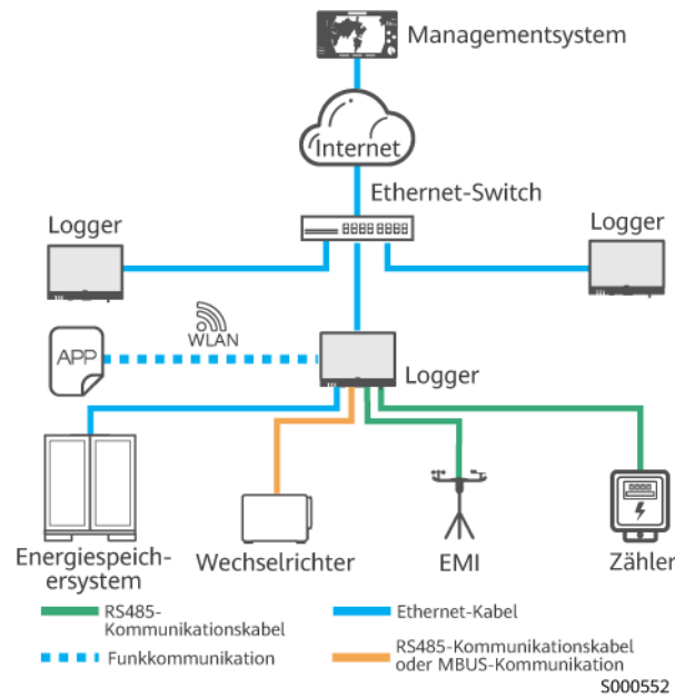
Abbildung 2-12 Ethernet-Sternnetzwerk
