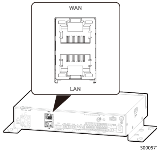
Abbildung 2-4 Ethernet-Anschlüsse
