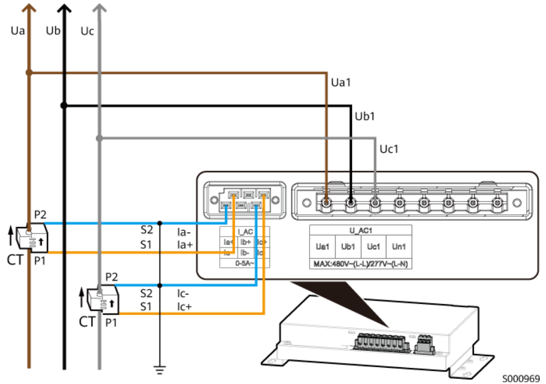
Abbildung 4-15 Schaltplan (Dreiphasen-Dreileiter)
