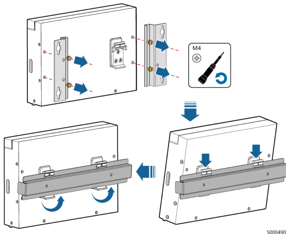
Abbildung 3-3 Installation auf einer Tragschiene
