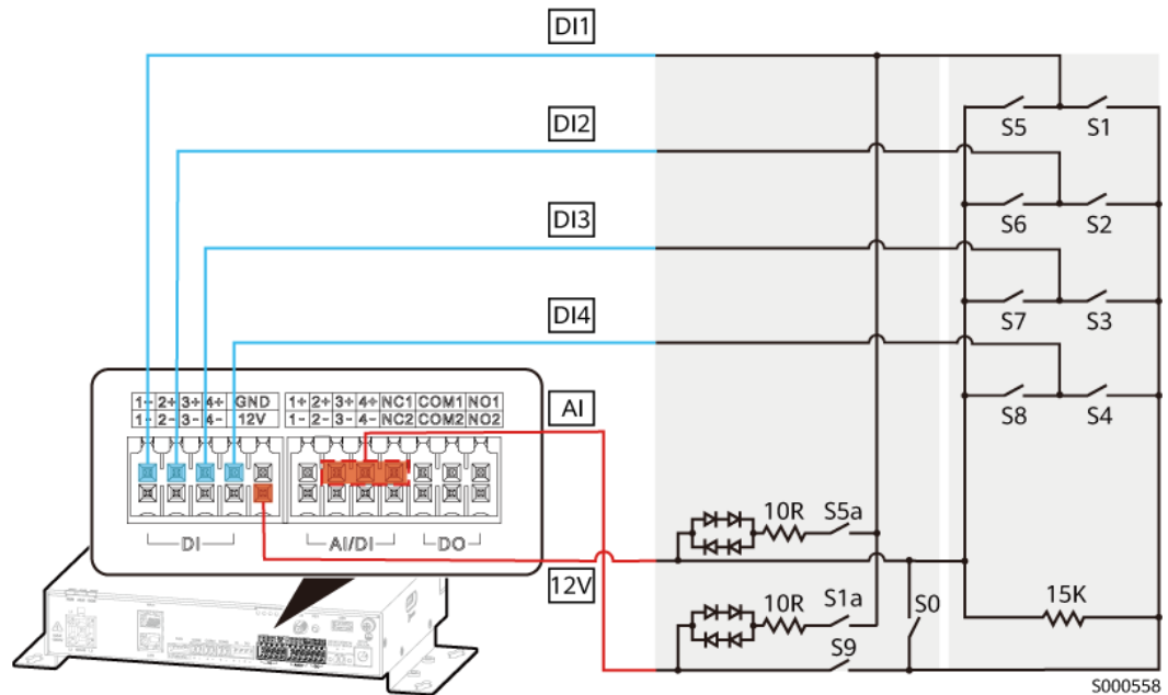
Abbildung 6-15 DRM-Kabelverbindung
