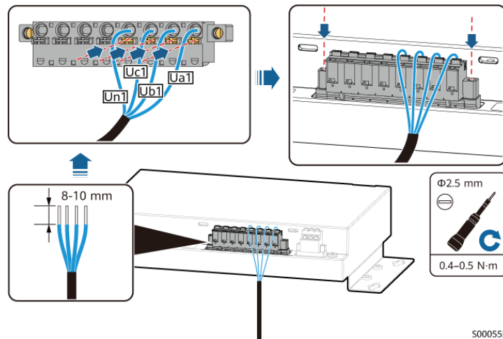
Abbildung 4-18 Anschließen eines Spannungserkennungssignalkabels
