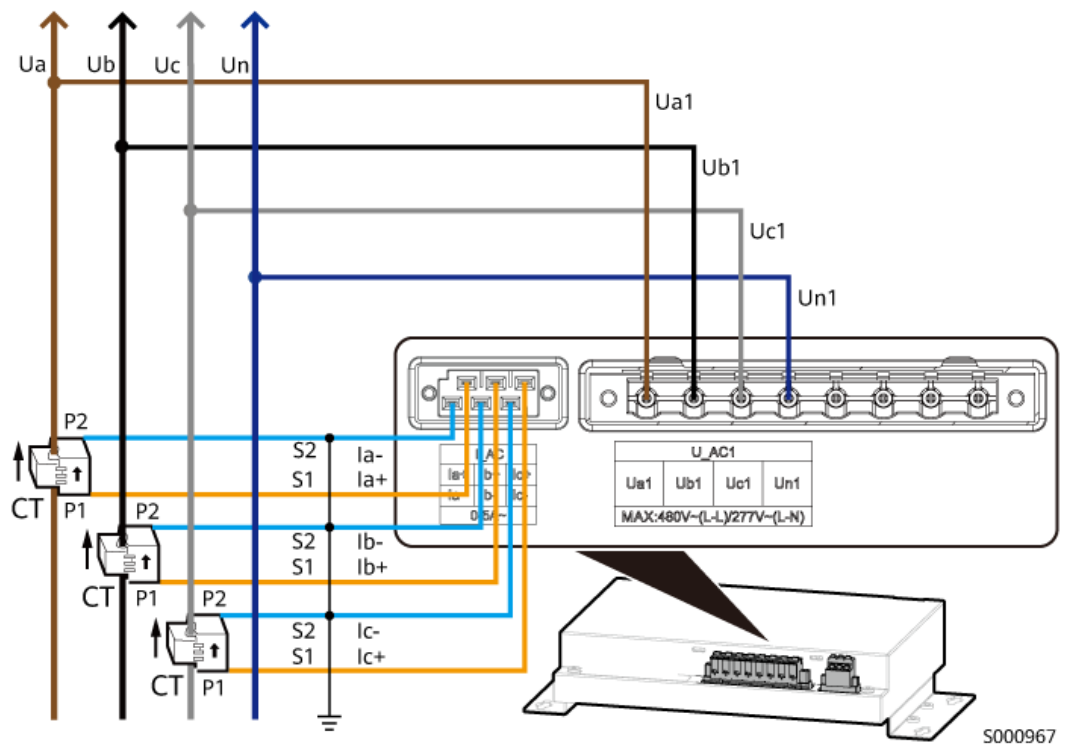
Abbildung 4-16 Schaltplan (Dreiphasen-Vierleiter)
