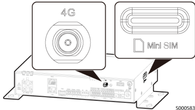
Abbildung 2-8 4G/SIM-Anschluss
