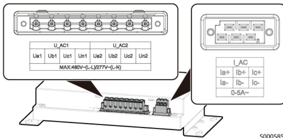
Abbildung 2-9 Strom-/Spannungserkennungsanschlüsse
