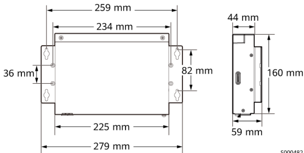
Abbildung 2-2 Produktabmessungen
