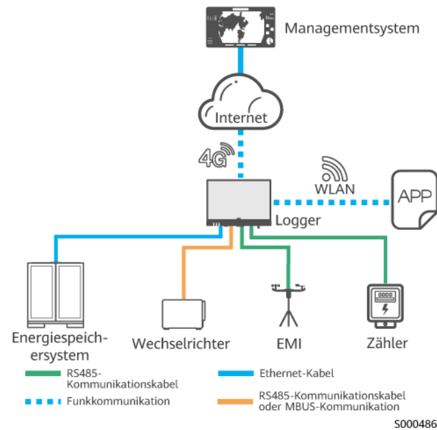
Abbildung 2-13 4G-Netzwerk
