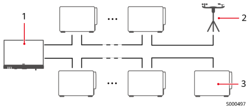
Abbildung 4-9 Kaskadenverbindung
