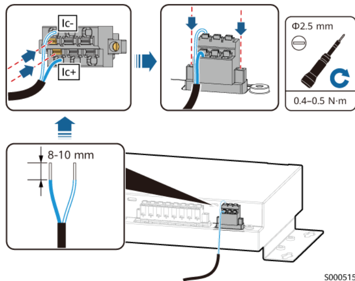
Abbildung 4-17 Anschließen eines Stromerfassungs-Signalkabels
