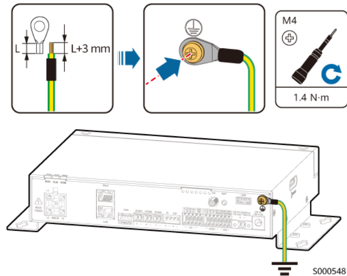
Abbildung 4-3 Anschließen eines PE-Kabels
