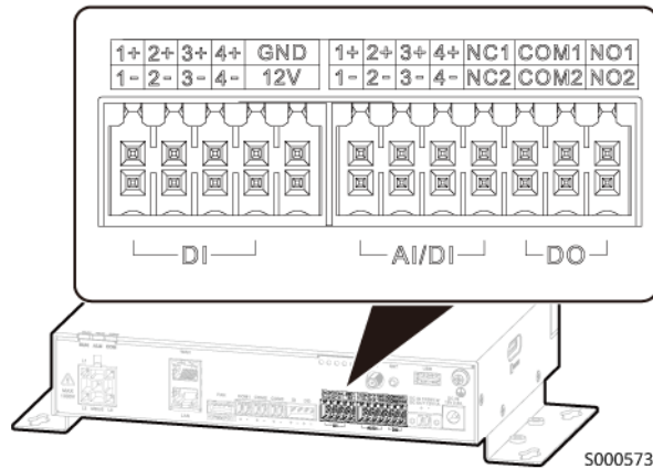
Abbildung 2-5 DI/DO/AI-Anschlüsse
