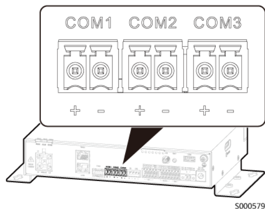
Abbildung 2-6 COM-Anschlüsse
