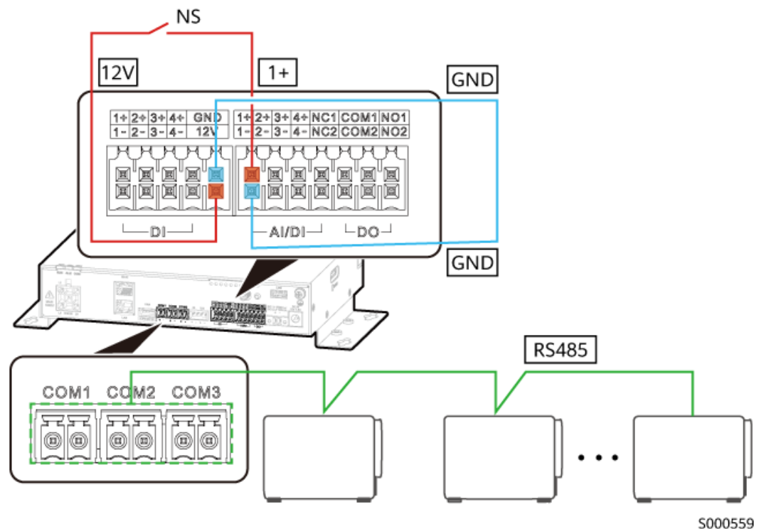
Abbildung 6-16 Vernetzungsplan
