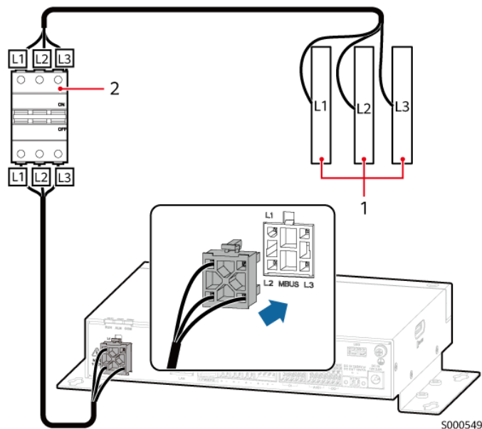
Abbildung 4-6 Anschließen eines MBUS-Kabels
