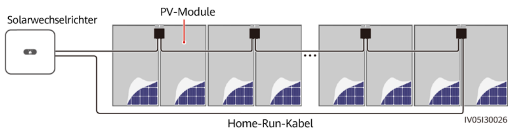
Abbildung 3-13 Verbotenes Kabelverlegung
