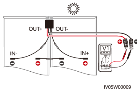
Abbildung 3-10 Messen der Ausgangsspannung eines Optimierers
