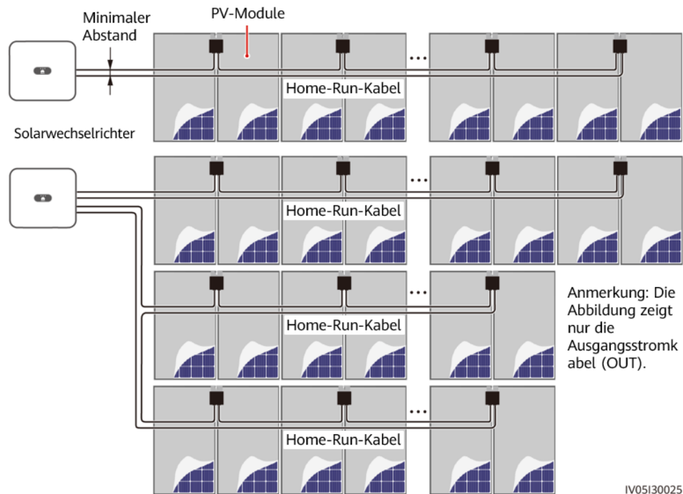
Abbildung 3-12 Erforderliches Kabelverlegung
