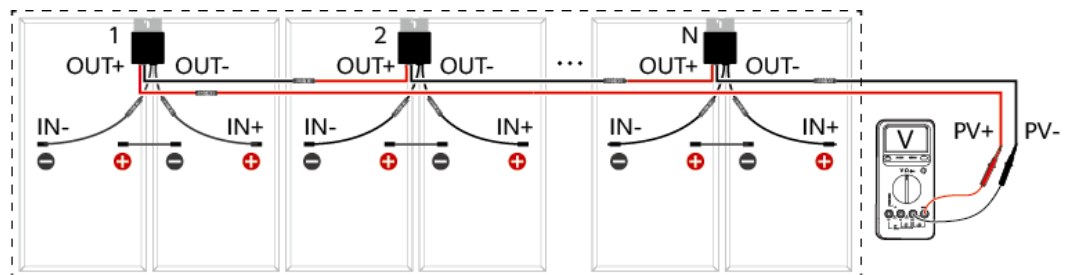
Abbildung 3-11 Messen der PV-String-Spannung
