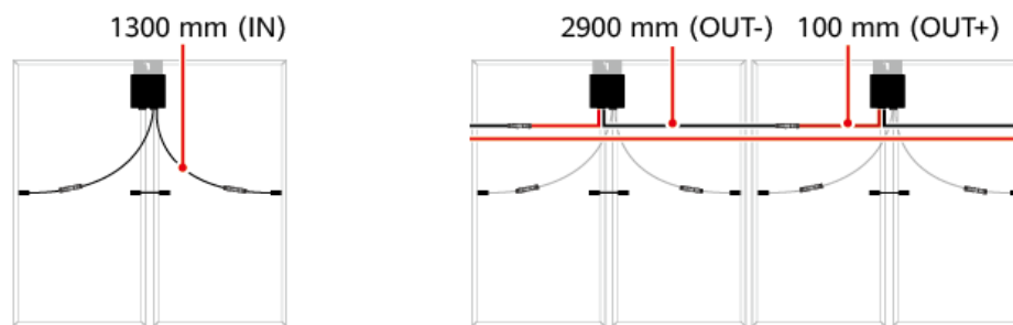
Abbildung 3-3 Optimierer mit langen Eingangsstromkabeln
