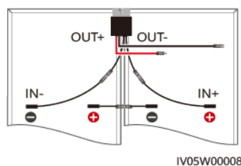
Abbildung 3-9 Anschließen des Optimierereingangs
